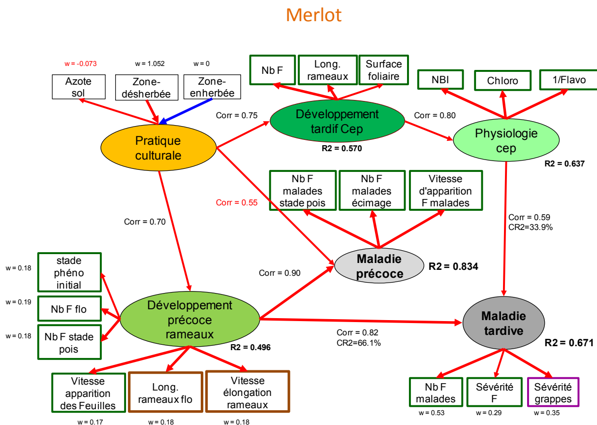
Figure 3 : Schéma de PLS-path least square pour la variété Merlot décrivant les relations entre l'environnement « Crop management », la croissance des ceps « Shoot growth early » et « Vine growth late », leur caractérisation physiologiques « Vine Physiology » et la maladie en début de saison « Disease early » et en fin de saison « Disease late ».
