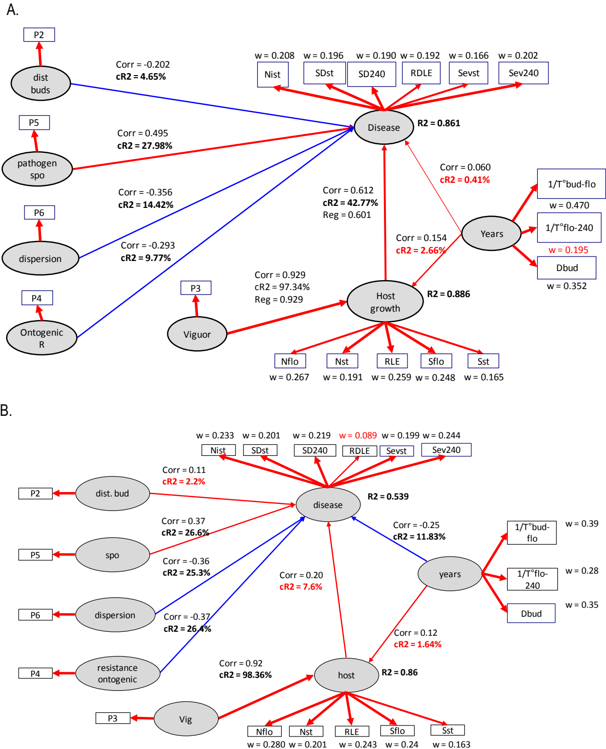
Figure 7 : Schéma de PLS path modèle issu de l'analyse de sensibilité décrivant les relations entre les variables latentes croissance de la plante « host growth », scénarii climatiques « years », « résistance ontogénic », « dispersion », sporulation « spo », distance entre les bourgeons « dist bud », vigueur « Vig ». Corr, indique le coefficient de corrélation, cR^2 la contribution relative des variables exogènes à la variable endogène, R^2 , le coefficient de régression entre deux variables latentes et w les poids des variables manifestes à la variable latente. A. Contamination précoce au stade 1 feuille, B. Contamination tardive au stade 4 feuilles. (en rouge les valeurs non significatives).
